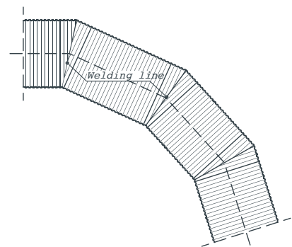
Fig. 6. Kromming van constructie - bovenaanzicht
