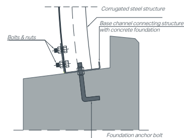
Fig. 8. Aansluiting van de staalconstructie op betonnen funderingen
