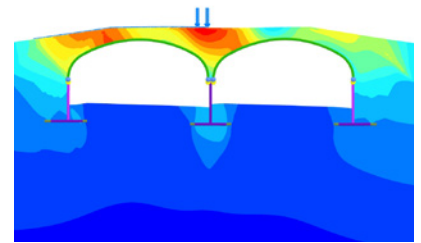
Fig. 2. Finite Element Method (FEM) model voor dubbele constructie
