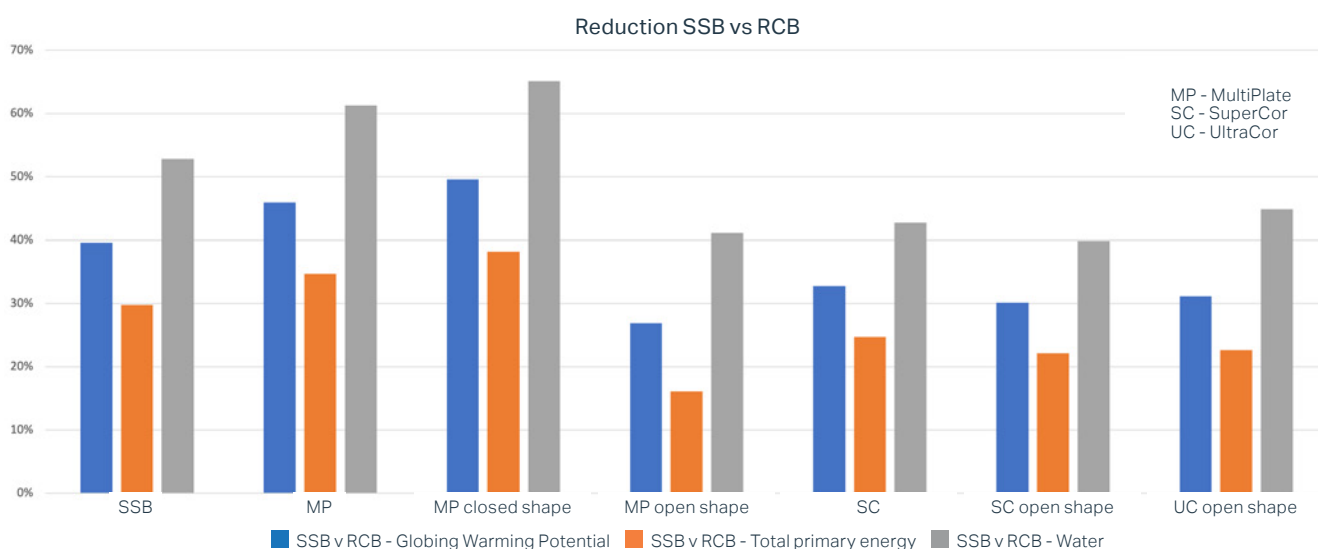
Fig. 2. LCA-analyse met vergelijking tussen grond-staalbruggen (soil-steel bridge - SSB) met gegolfde stalen constructie en bruggen van gewapend beton
